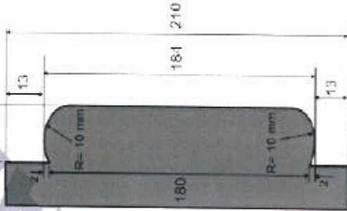
SUAJE PARA FORMAR SEGURO EN SOLAPA DE LA CARA FRONTAL
