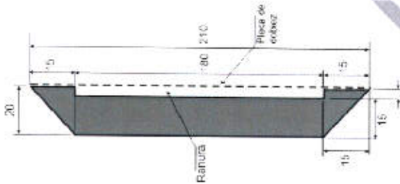
SUAJE PARA FORMAR RANURA EN SOLAPA DE CARA LATERAL
